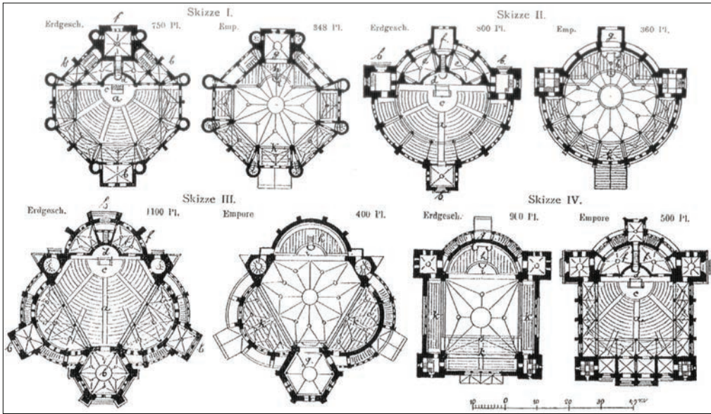
7. Схемы протестантских кирх. Йоганес Отцен. «Висбаденская программа».
