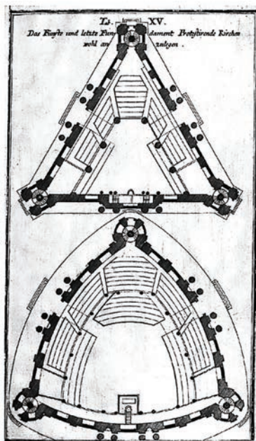
6. Проект треугольной кирхи Л. К. Штурма, 1718 г.
